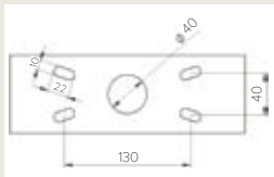
Platine de fixation
